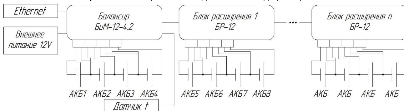
Рисунок 7.2 – схема подключения модификации PRO
