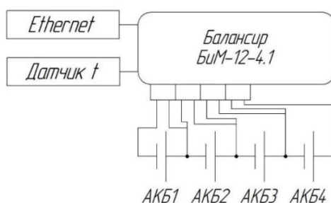
Рисунок 7.1 – общая схема подключения модификации BASIC
